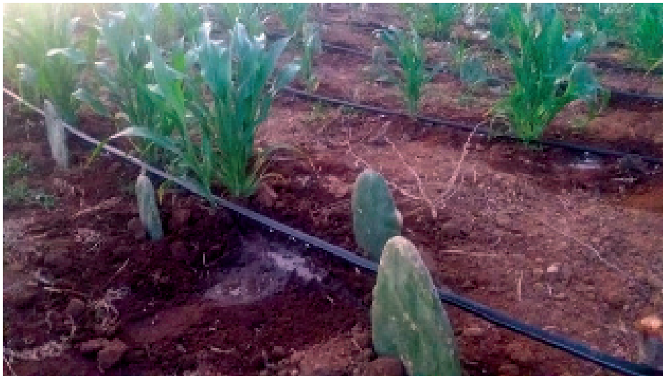
Figura 11 - Detalhe do sistema de irrigação por gotejamento. Fonte: Acervo PROCASE.
