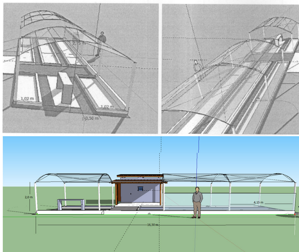
Figura 34 - Projeto de engenharia dos viveiros implantados pelo PROCASE. Acima: Versão mal concebida e que gerou prejuízos as ações de viveiricultura. Abaixo: Ajustes do projeto que permitiram a retomada da iniciativa e o sucesso de algumas ações. Fonte: Setor de Engenharia PROCASE.
