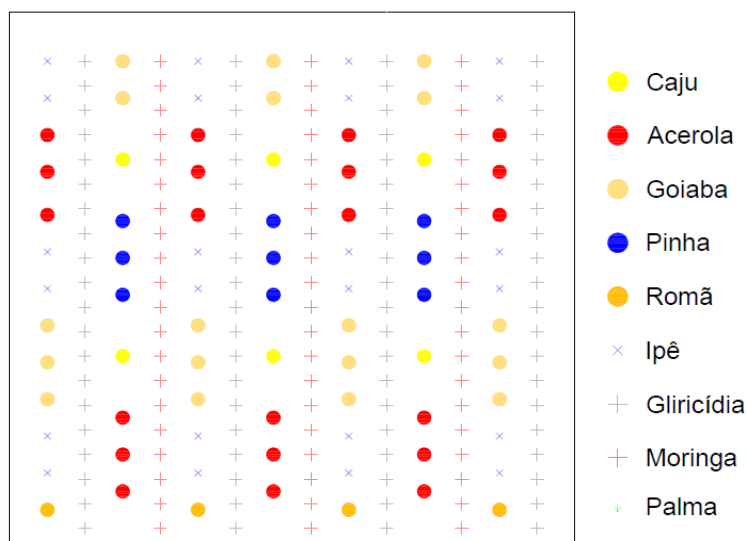
Figura 22 - Área conceitual de plantio dos SAF. Dimensões de 35 x 35 m (1.225 m 2 ). Fonte: PROCASE & FLOREST (2018a).
